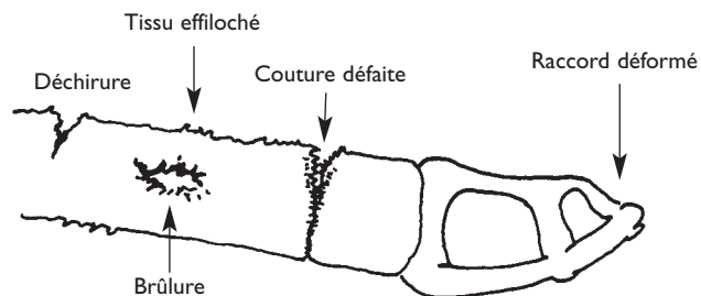
Figure 3.7 Inspection des élingues de fibres synthétiques
