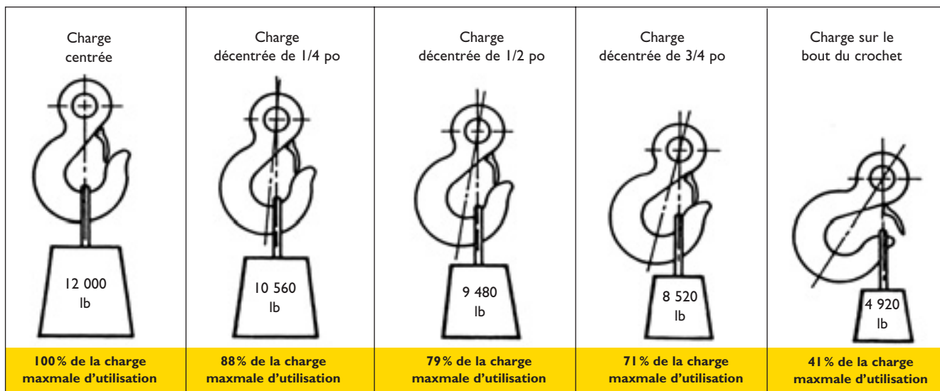
Figure 3.14 Tension dans la gorge d'un crochet d'une capacité de 12 000 lb.
