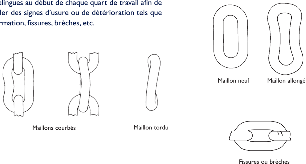
Figure 3.5 Inspection d'une élingue de chaîne
