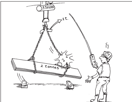
Deux élingues d'une capacité d'une tonne sont utilisées pour lever une charge de deux tonnes. Une des élingues casse.
