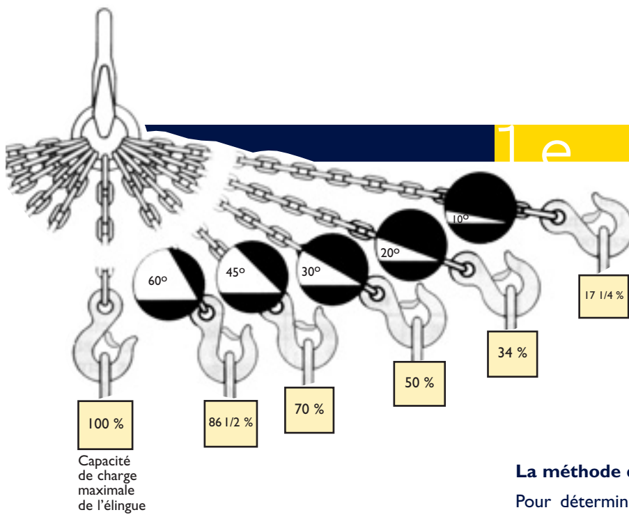
Figure 3.34 Réduction des charges maximales en fonction de l'angle
