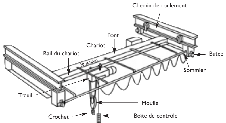
Figure 2.2 Composantes d'un pont roulant
