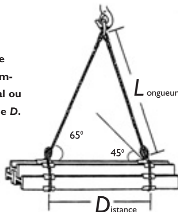
Figure 3.35 Longueur des élingues et points d'attache
