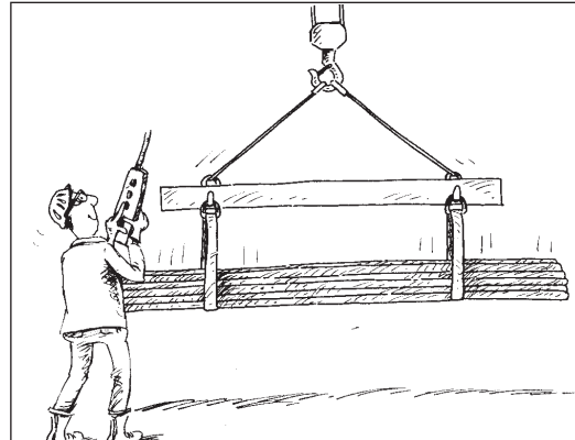
L'opérateur utilise un palonnier ou encore des élingues de longueur appropriée.
